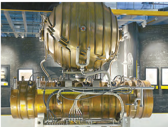
大型正負電子（LEP）對撞機加速腔。
